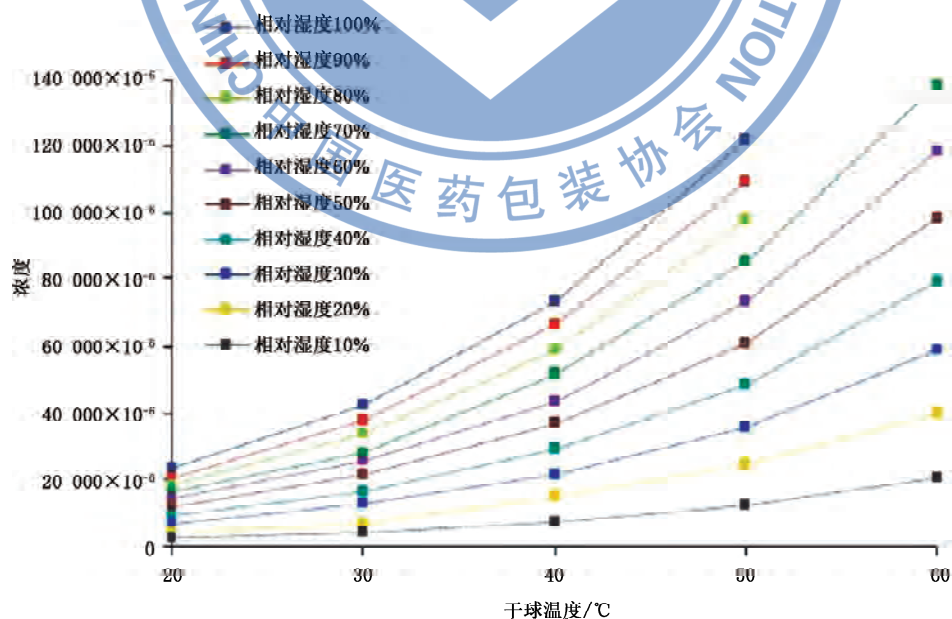
图 A.1 水在空气中的浓度作为温度与相对湿度函数关系的示例
